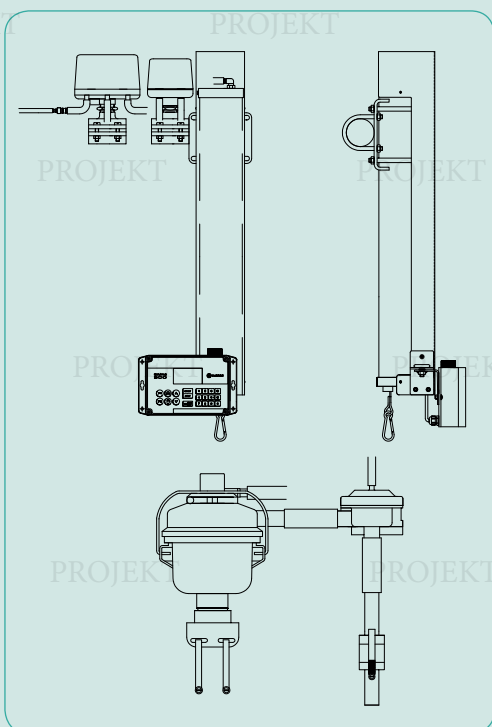
PLŪSMAS MĒRĪTĀJS
